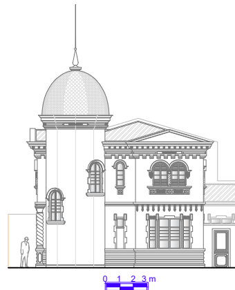
Elevação 02
