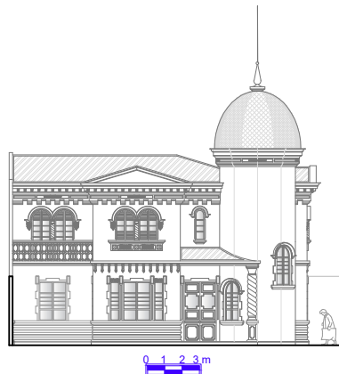
Elevação 01
